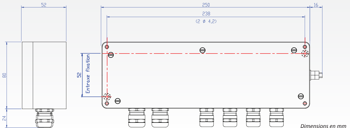
Schéma boîtier aluminium
